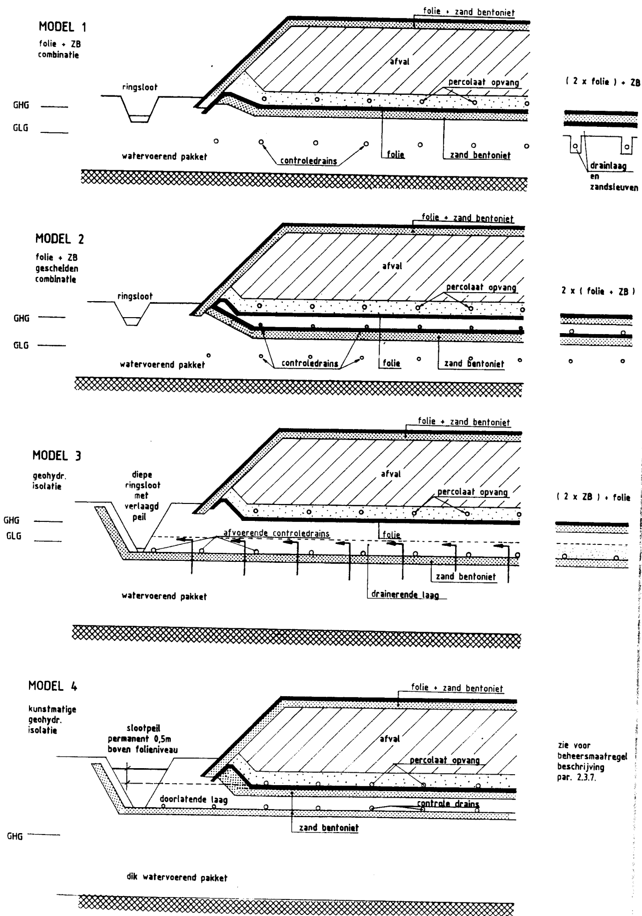
figuur 4 Onderafdichtingsconstructies
